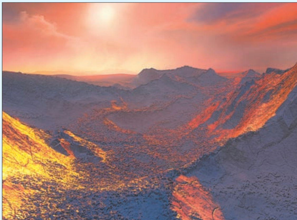
FOTO:ESO-M. Kornmesser / Imatge de la nova "superterra freda" descoberta al voltant de l'estrella de Barnard
