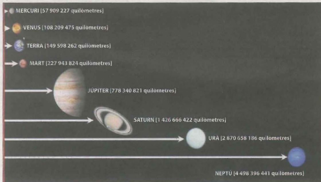
Distàncies mitjanes en quilòmetres dels planetes del Sistema Solar respecte del Sol.
